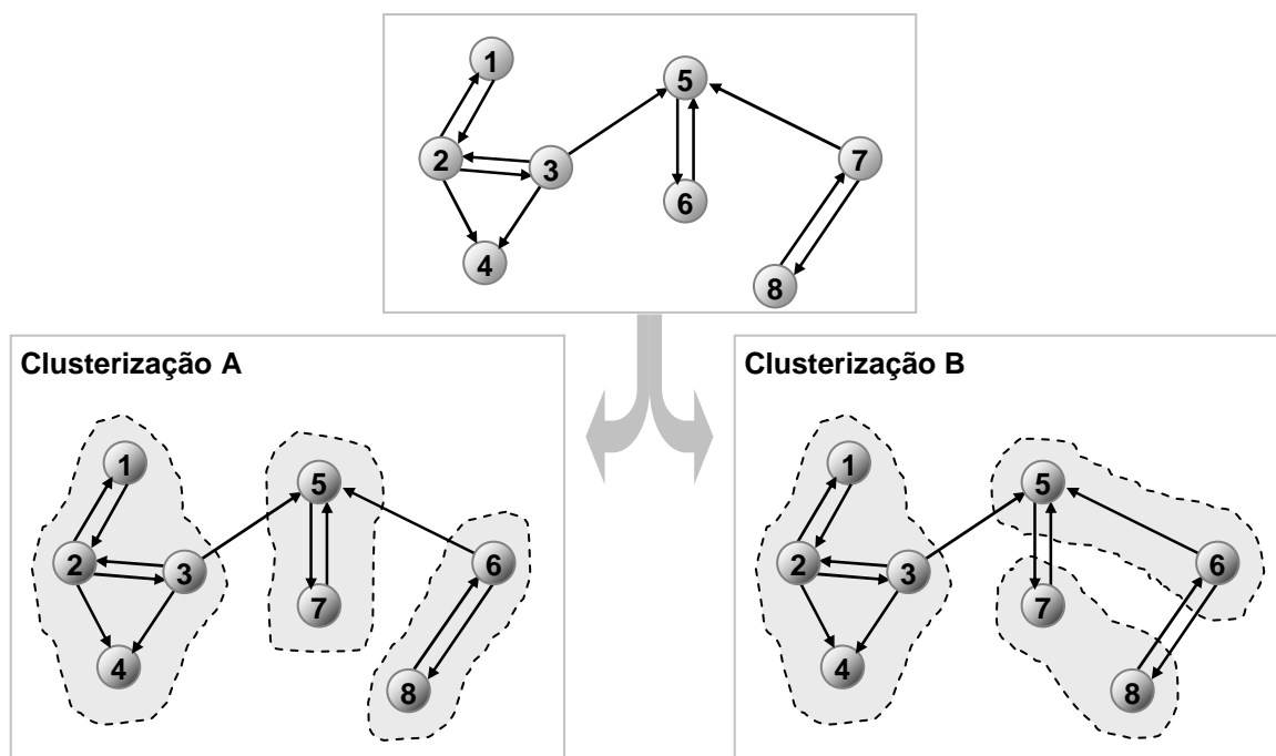
Figura 3.2 – Exemplos de clusterização de um grafo orientado com 8 vértices [12]
